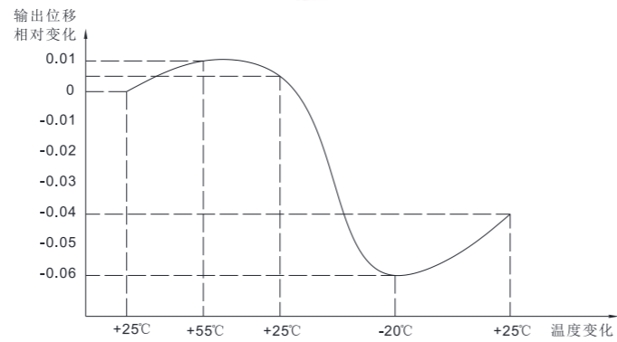
高低温变化测试曲线
